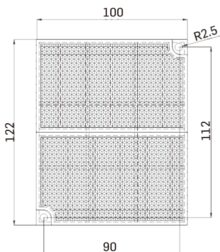
Fig.10a(unit: mm)
